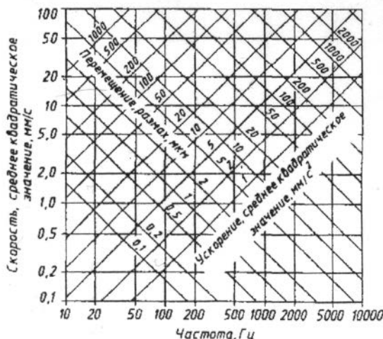
Рисунок А1 — График, указывающий соотношение между ускорением, скоростью и перемещением для гармонической вибрации
